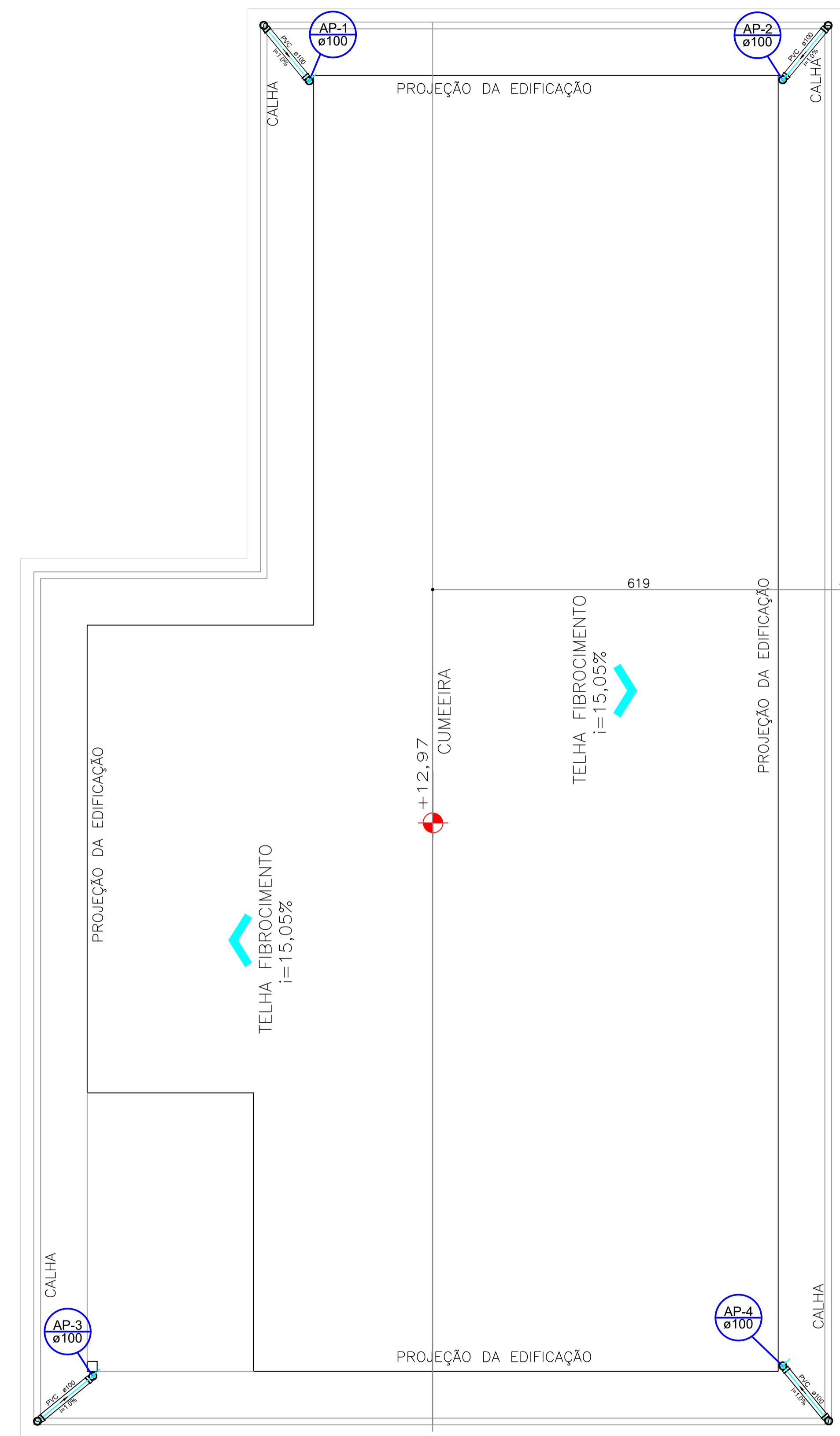
PLANTA DE COBERTURA ESCALA 1:50
