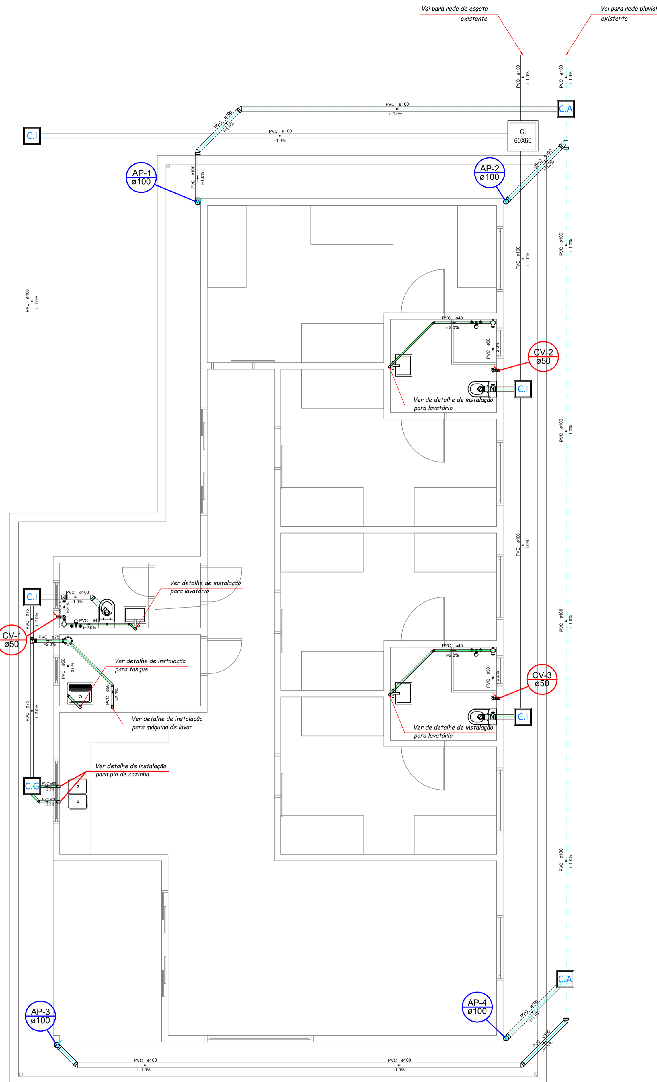
PLANTA BAIXA CASA 10 - ESGOTO ÁREA TOTAL COMPUTÁVEL: 173,74m 2 ESCALA 1:50
