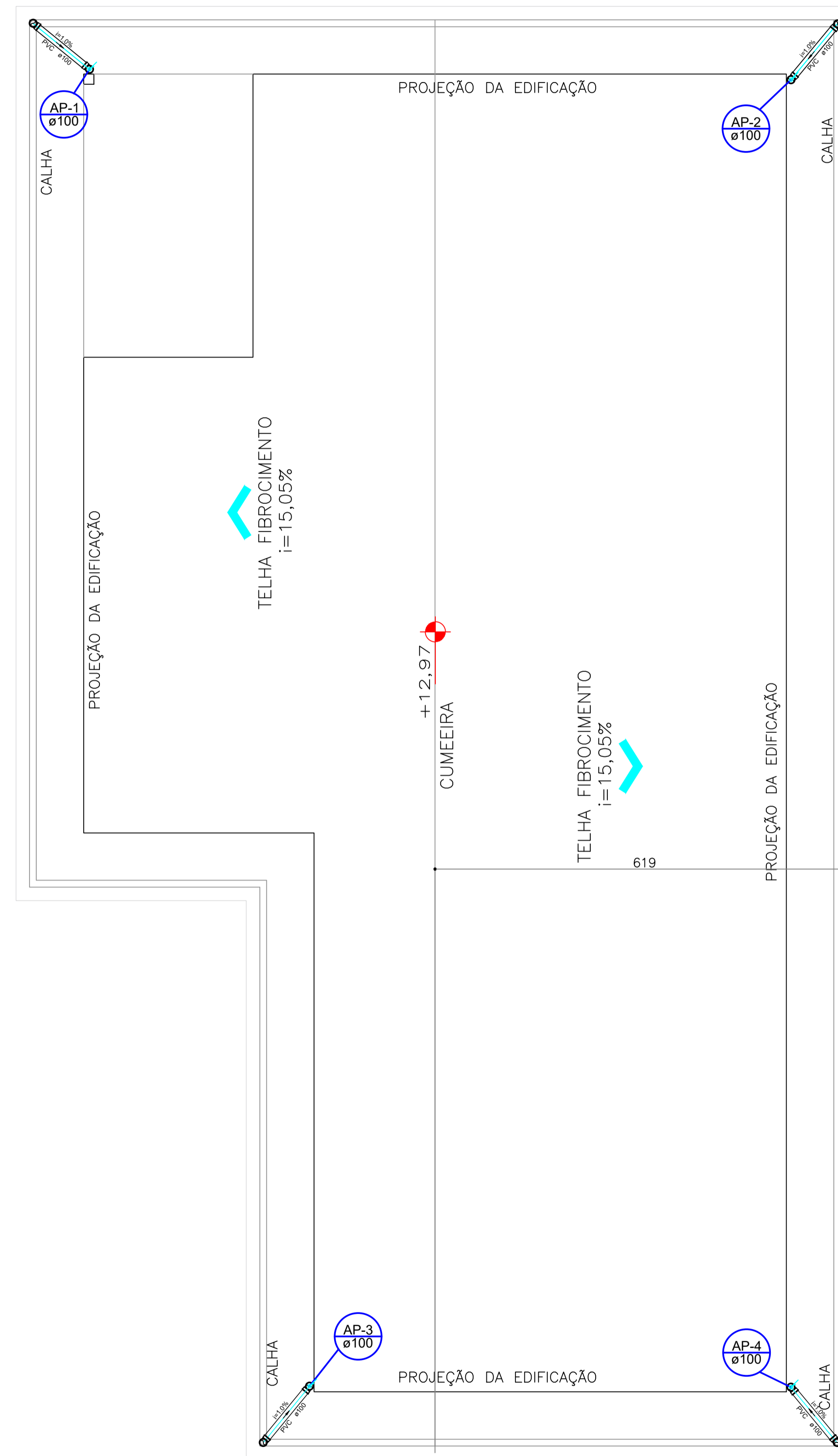
PLANTA DE COBERTURA ESCALA 1:50
