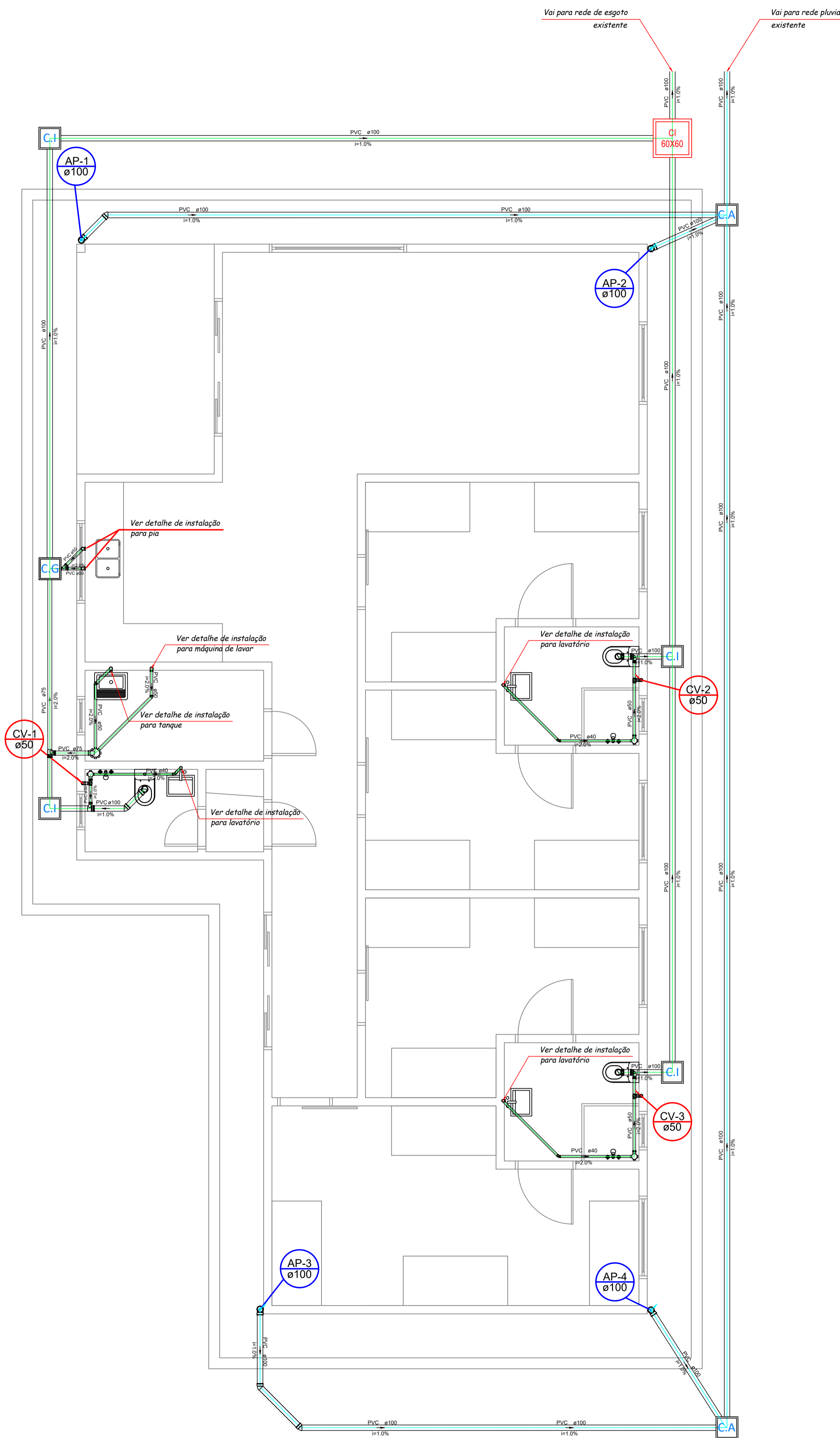
PLANTA BAIXA CASA 11 - ESGOTO ÁREA TOTAL COMPUTÁVEL: 173,74m 2 ESCALA 1:50
