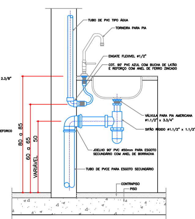
DETALHE PIA DE COZINHA Esc: 1/10
