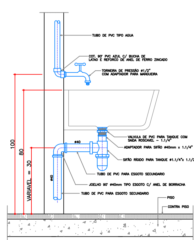
DETALHE TANQUE Esc: 1/10
