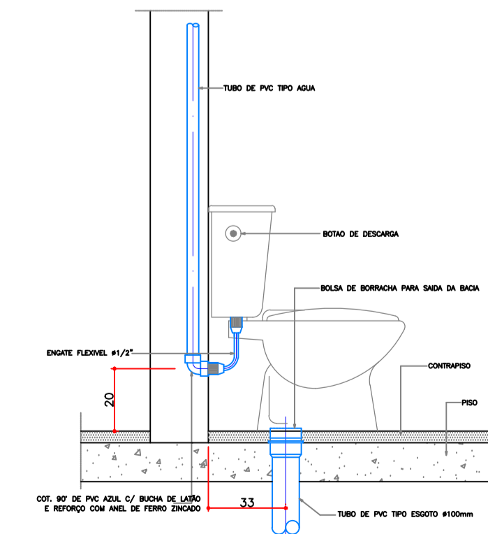
DETALHE VASO SANITÁRIO Esc: 1/10
