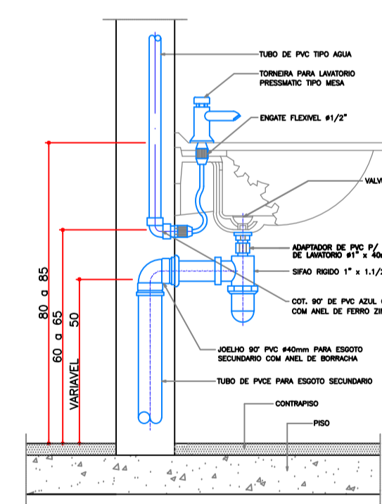
DETALHE LAVATÓRIO Esc: 1/10
