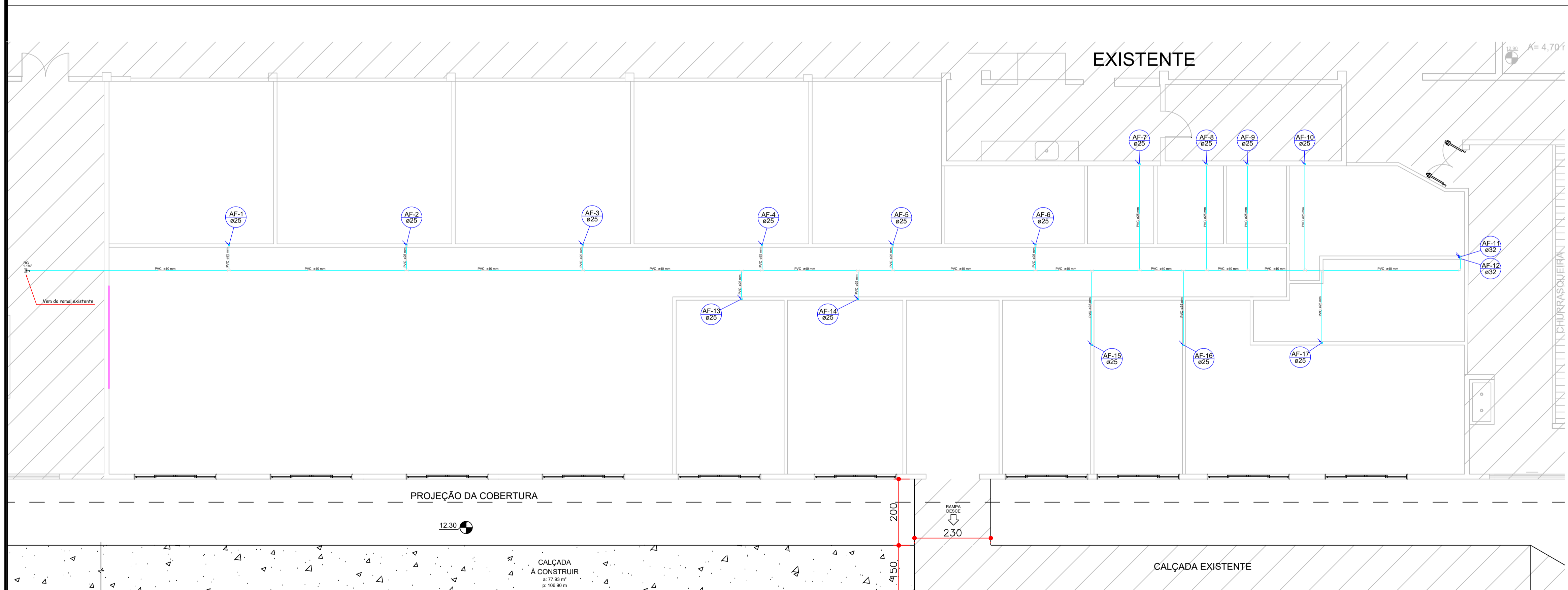
PLANTA BAIXA DISTRIBUIÇÃO (NÍVEL RESERVATÓRIO) - ÁGUA FRIA ÁREA TOTAL: 454,44m 2 ESC. 1/50
