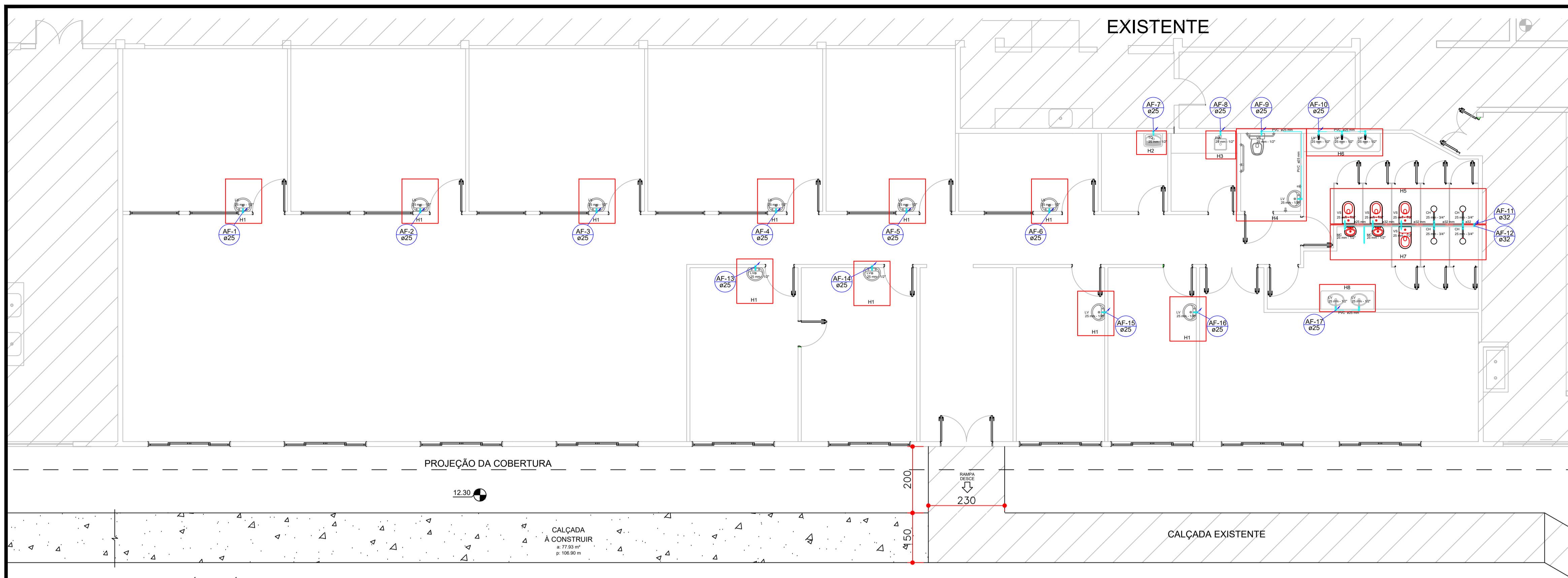
PLANTA BAIXA TÉRREO - ÁGUA FRIA ÁREA TOTAL: 454,44m 2 ESC. 1/50
